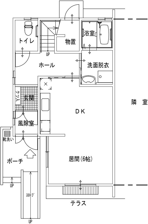
1階 平面図
