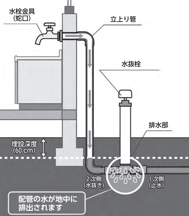
▲不凍水栓の水抜きの仕組み
