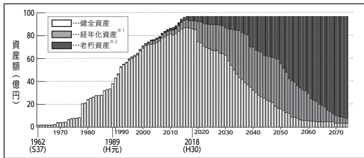
【図】本町の水道施設の健全度
