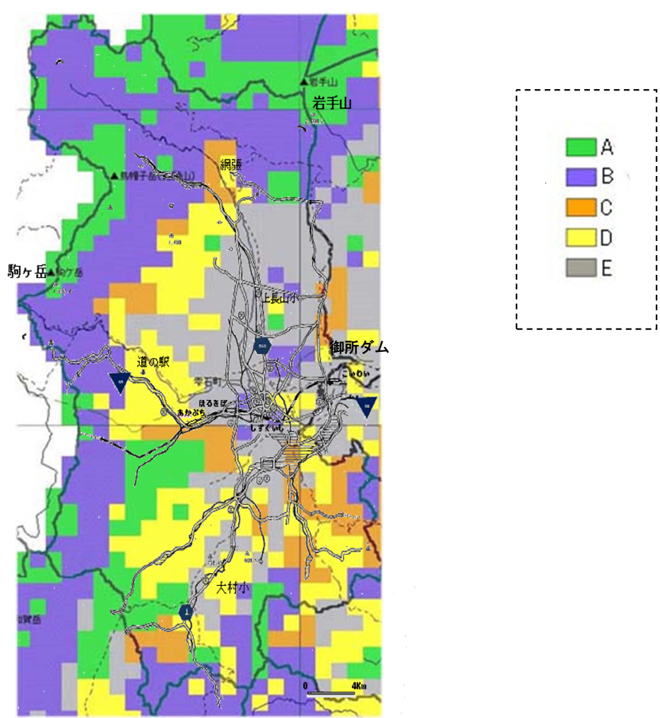
参考資料 図4 生物的環境評価図 (岩手県自然環境保全指針 抜粋)
