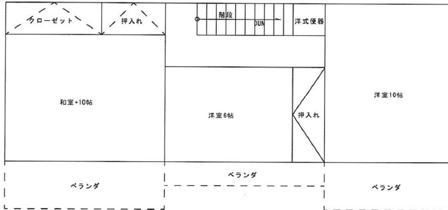
2階平面図
