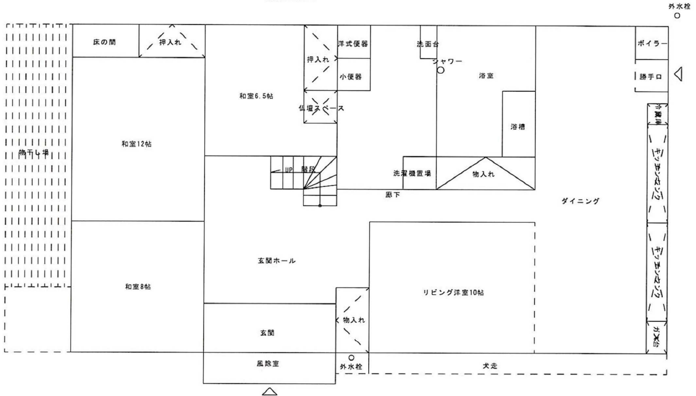
1階平面図
