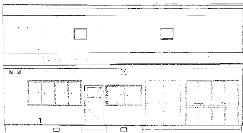
东侧 立面图 S=1:50
