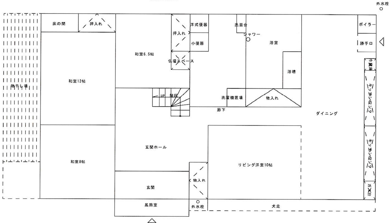
1階平面図
